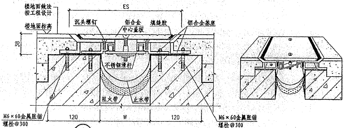
图 7 变形缝构造示意图
